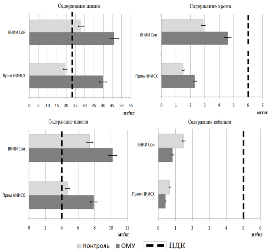
Рис. 1 Содержание Zn, Cr, Ni и Co в почвах исследуемых агрохимических стационаров относительно норм ПДК, мг/кг
