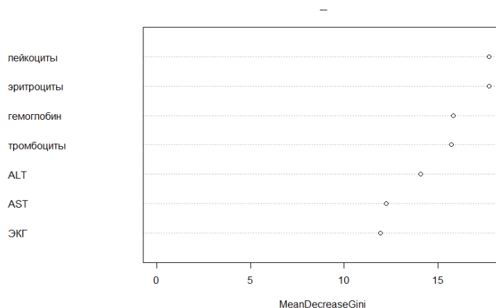
Рис. 2. Степень важности предикторов
