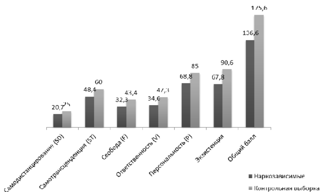
Рис. 1. Средние значения наркозависимых и контрольной выборки
