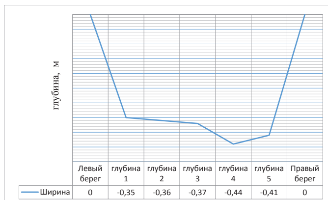
Рисунок 2 - Поперечный профиль водного сечения р. Светлогорки
