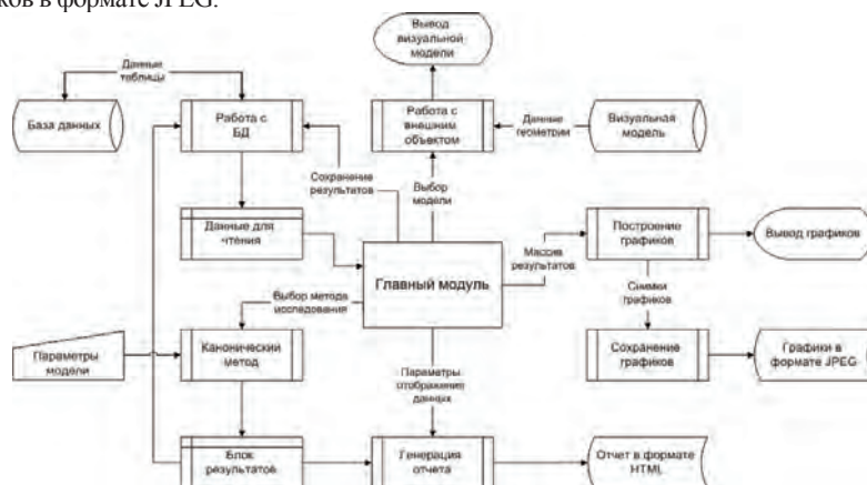
Рисунок 1 - Функциональная схема ВПК
