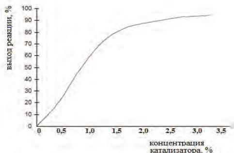
Рис.2. Влияние концентрации катализатора на выход реакции, при температуре кипения смеси веществ.
