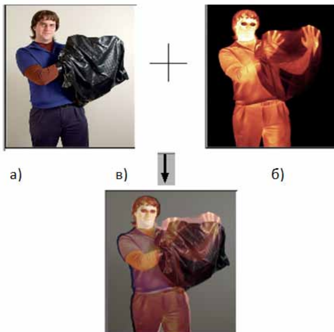
Рисунок 4 - а) ТВ изображение, б) ИК изображение, в) совмещенное изображение
