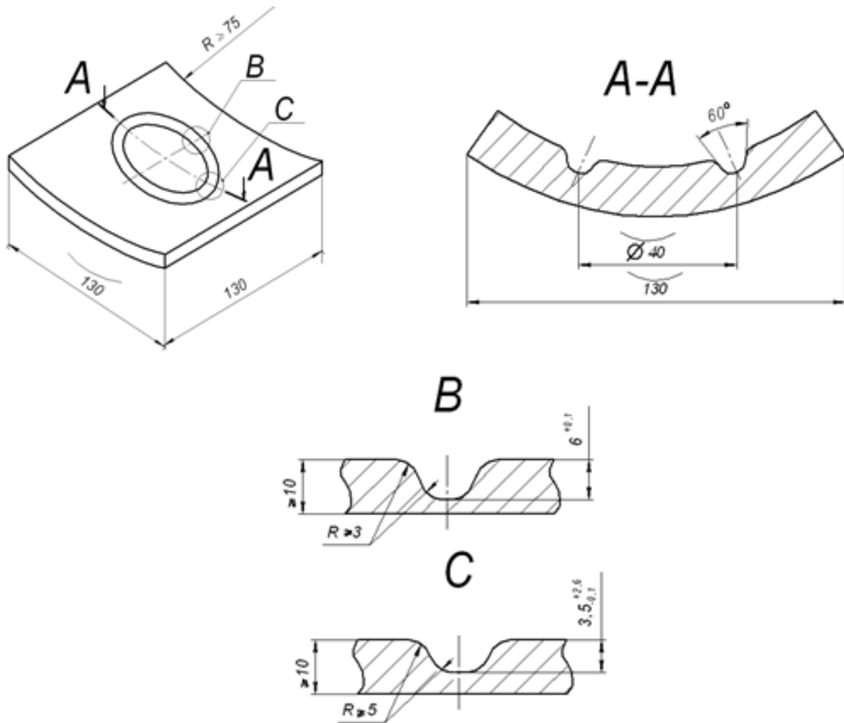
Рисунок 2 - Образец для испытания на горячие трещины при сварке участков металла, обращенных при эксплуатации к рабочей среде
