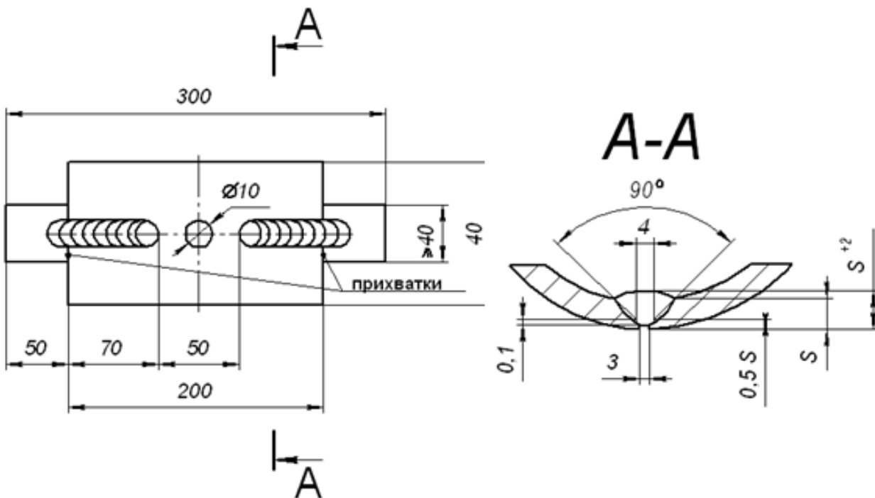
Рисунок 3 - Образец для испытания на горячие трещины при сварке поверхности трубного элемента, обращенного при эксплуатации к рабочей среде
