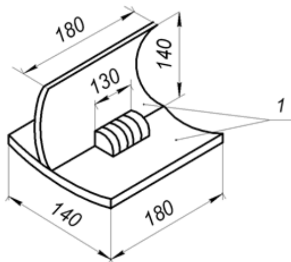
Рисунок 1 - Наплавка валика при односторонней сварке таврового образца после эксплуатации:
