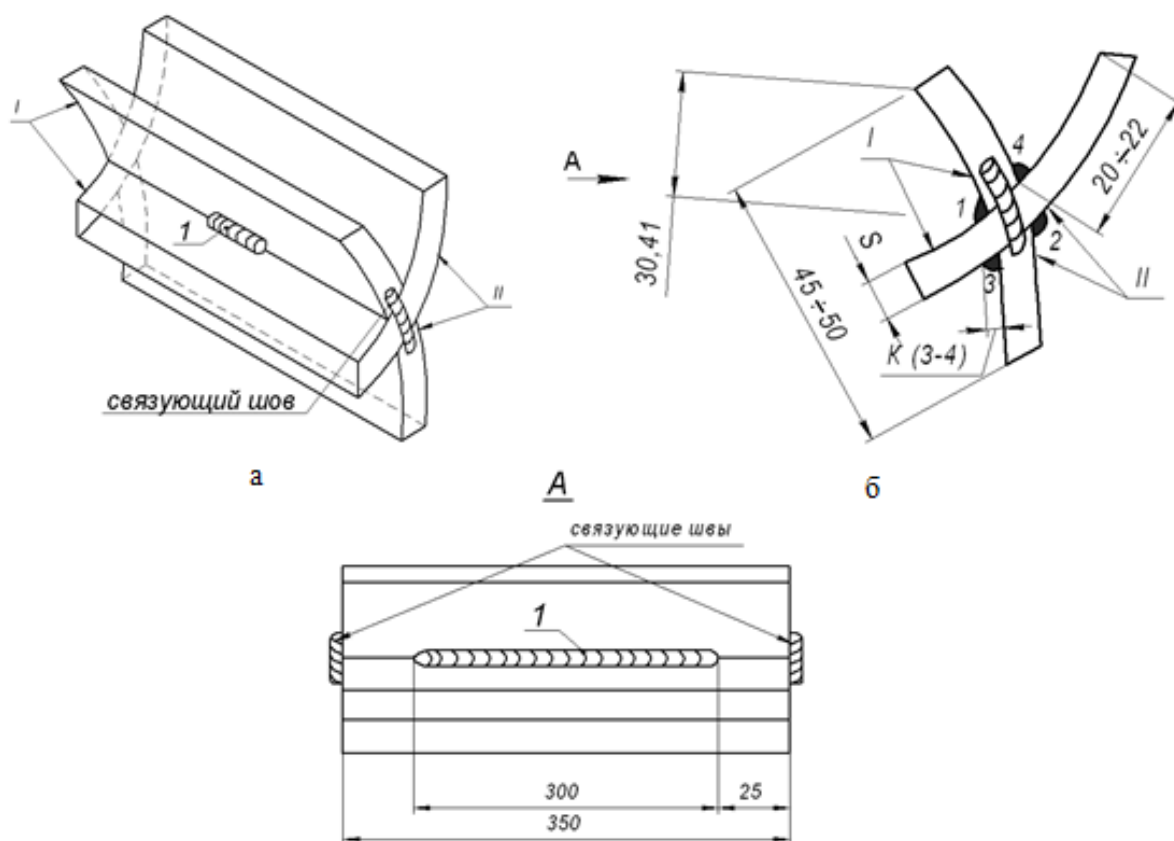
Рисунок 4 - Образец для испытания на холодные трещины при сварке (тип VII ГОСТ 26388):
