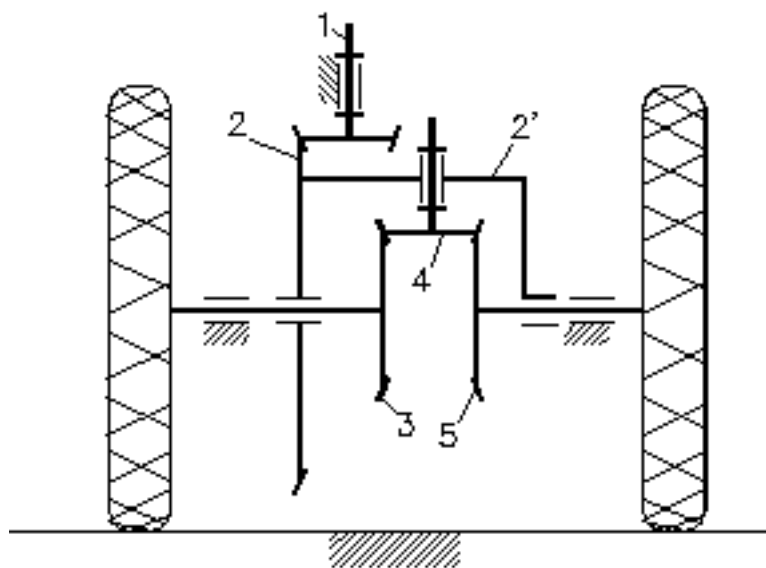
Рис. 2. Автомобильный дифференциал
