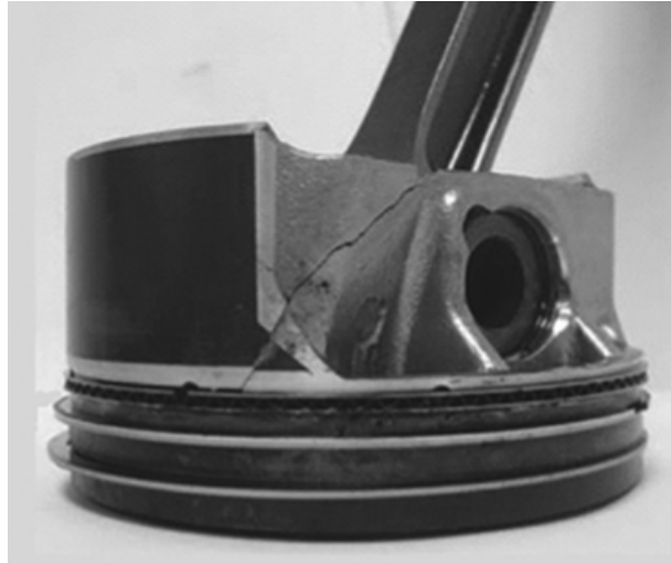
Рис. 1 – Трещина на поршне, возникшая в результате преждевременного воспламенения
