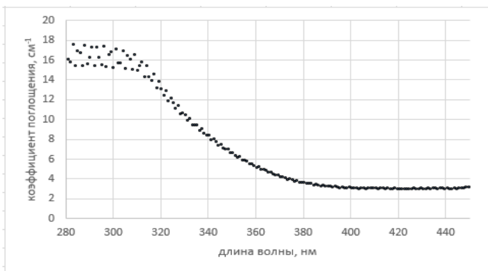
Рисунок 2 – График зависимости коэффициента поглощения от длины волны
