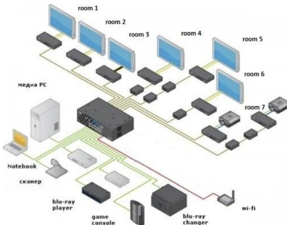
Рисунок 2 Система мультимедиа
