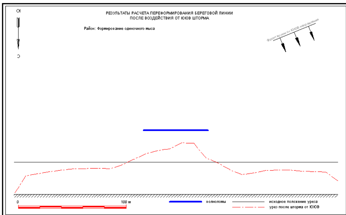
Рис. 4. Результаты моделирования формирования искусственного мыса при l = 20h_{cr} = 60 м, b = l
