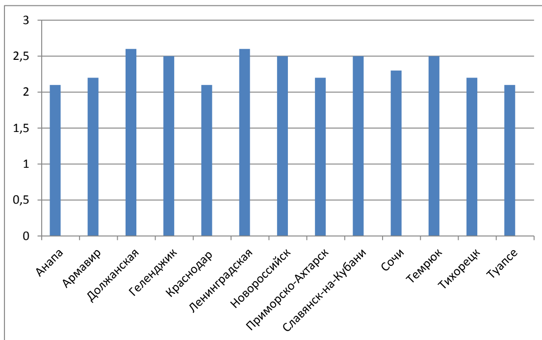
Рис. 2. Ежегодное уменьшение выбросов парниковых газов (тонн эквивалента CO 2 ) за счет устройства типовой мультифункциональной ТНУ для различных туристских дестинаций Краснодарского края
