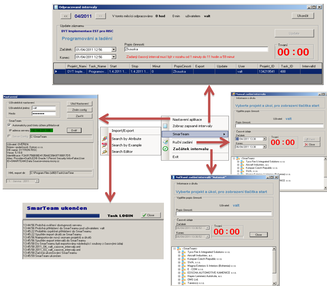
Figure 2 Module TaskUserTime
