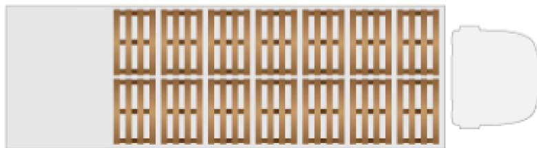
Рисунок 10– Схема размещения европаллетов в кузове SCANIA R400
