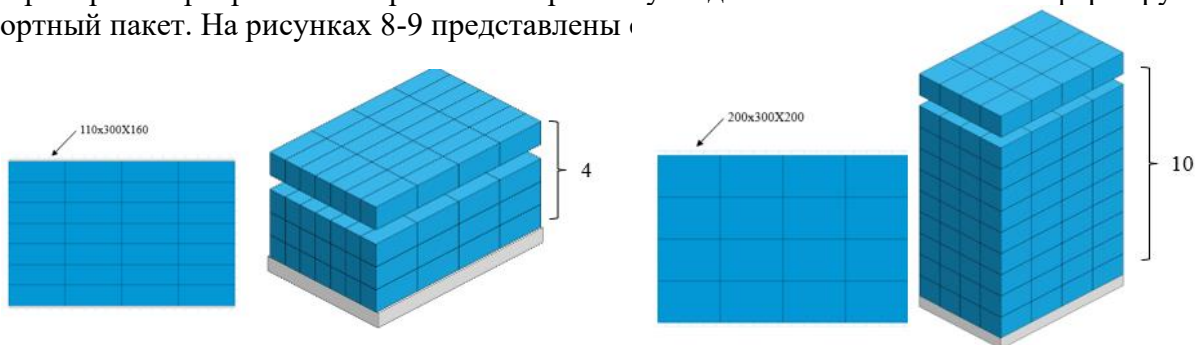
Рисунок 8 – Вариант укладки патронов 7,62x39 FMJ-1 и 5,6x39 ТПЗ FMJ на паллет
