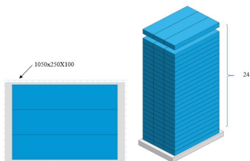
Рисунок 7 – Вариант укладки ТОЗ-78-04М на паллет
