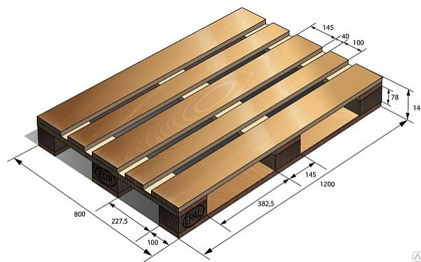
Рисунок 5 – Размеры европаллета
