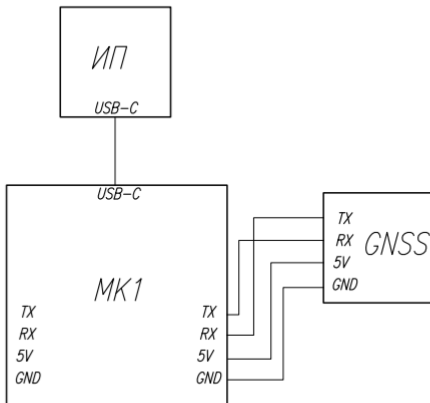
ИП – источник питания, MK1 – микроконтроллер Raspberry Pi 4b, GNSS – приемник L76K Waveshare
