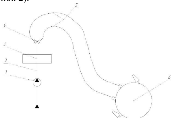
Рисунок 2 – Принципиальная схема установки
