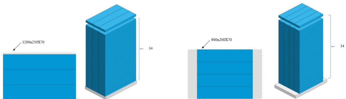
Рисунок 6 – Вариант укладки ТОЗ-34Р и КО ВСС на паллет
