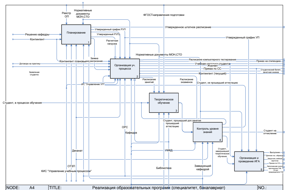
Рис.1. Пример использования нотации IDEF0
