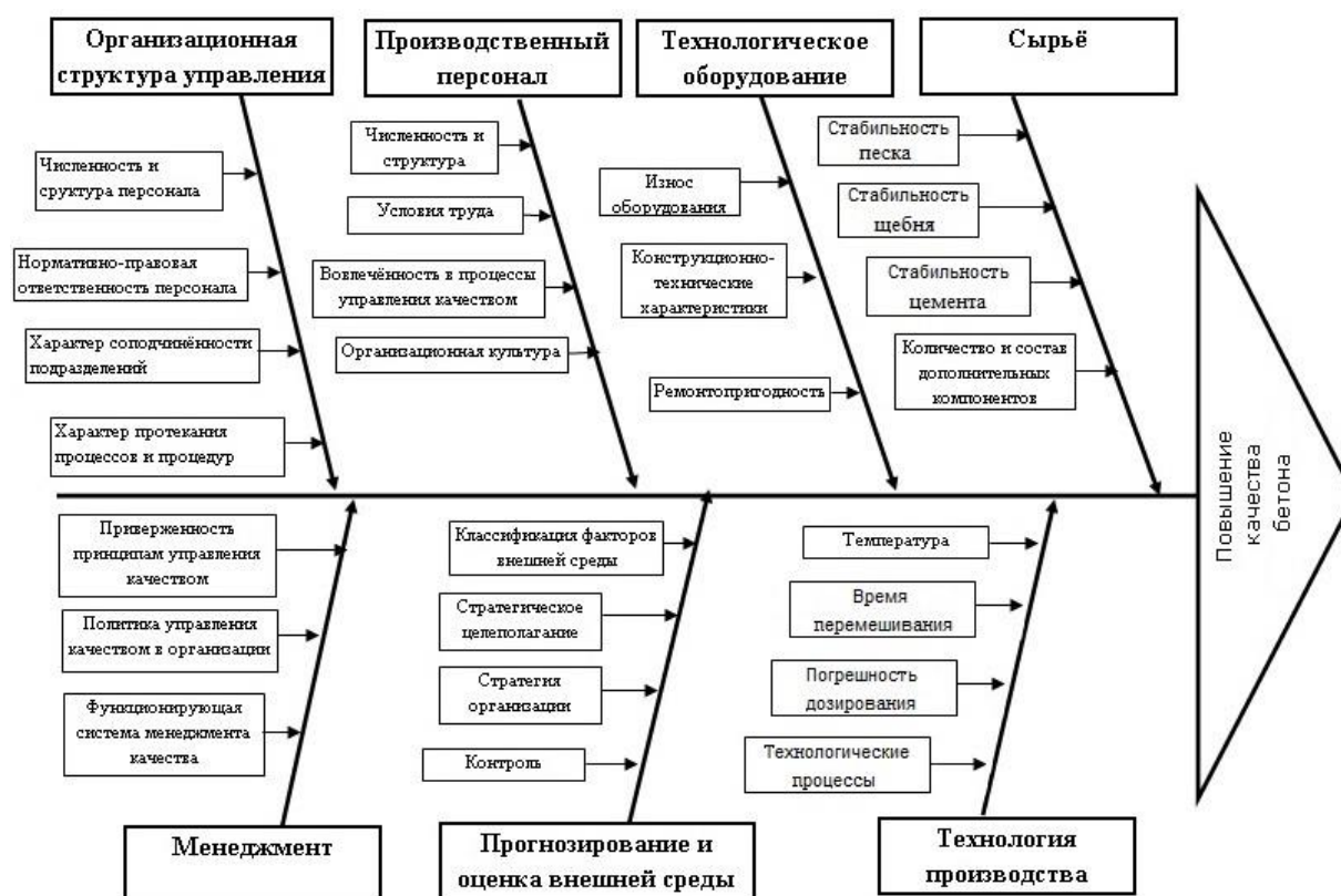
Рис. - Диаграмма Исикавы повышения качества бетона
