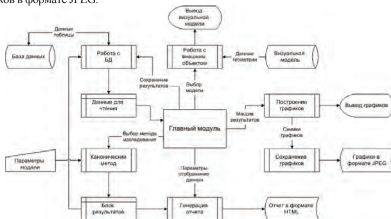
Рисунок 1 - Функциональная схема ВПК
