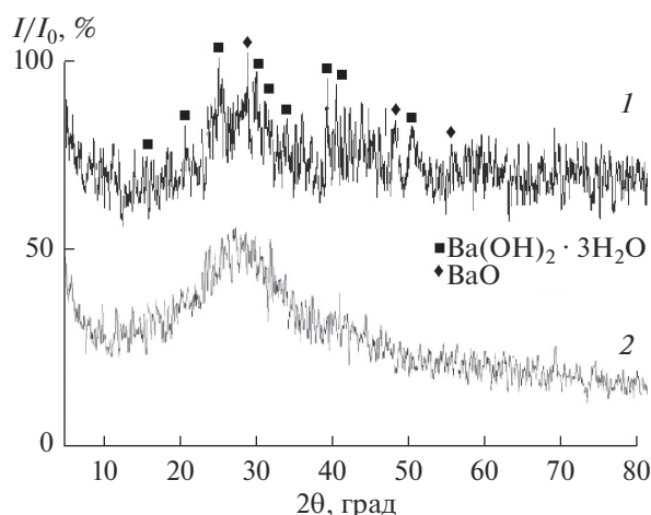
Рис. 1. Дифрактограммы образцов: 1 – \text{BaSiO}_3 \cdot 2.3\text{H}_2\text{O} ; 2 – \text{BaAl}_2\text{Si}_2\text{O}_8 \cdot 2.6\text{H}_2\text{O} .
