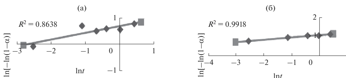
Рис. 8. Кинетика топохимических процессов сорбции ионов: а – кальция, б – стронция.
