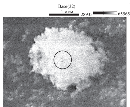
Рис. 5. СЭМ-изображение частиц образца \text{BaAl}_2\text{Si}_2\text{O}_8 \cdot 2.6\text{H}_2\text{O} .
