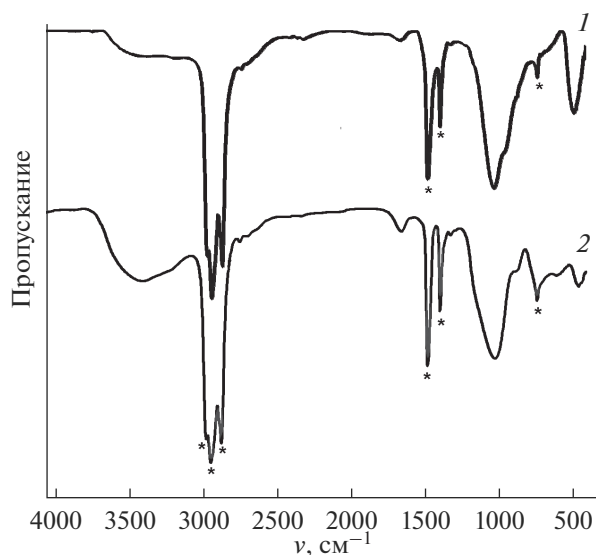
Рис. 2. ИК-спектры образцов: 1 – \text{BaSiO}_3 \cdot 2.3\text{H}_2\text{O} , 2 – \text{BaAl}_2\text{Si}_2\text{O}_8 \cdot 2.6\text{H}_2\text{O} (*пики вазелина).
