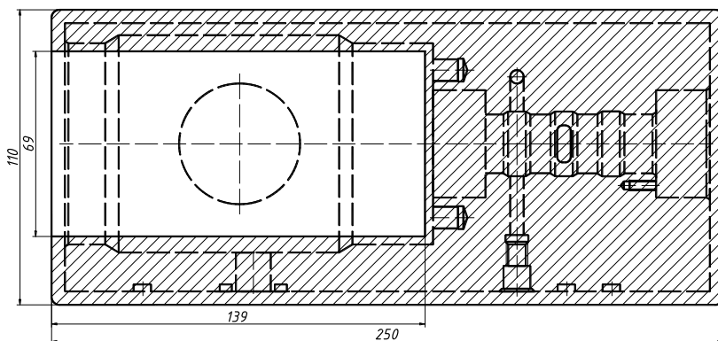
Рис. 1. Эскиз кованной поковки
