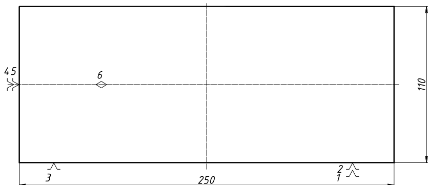
Рис. 2. Схема базирования
