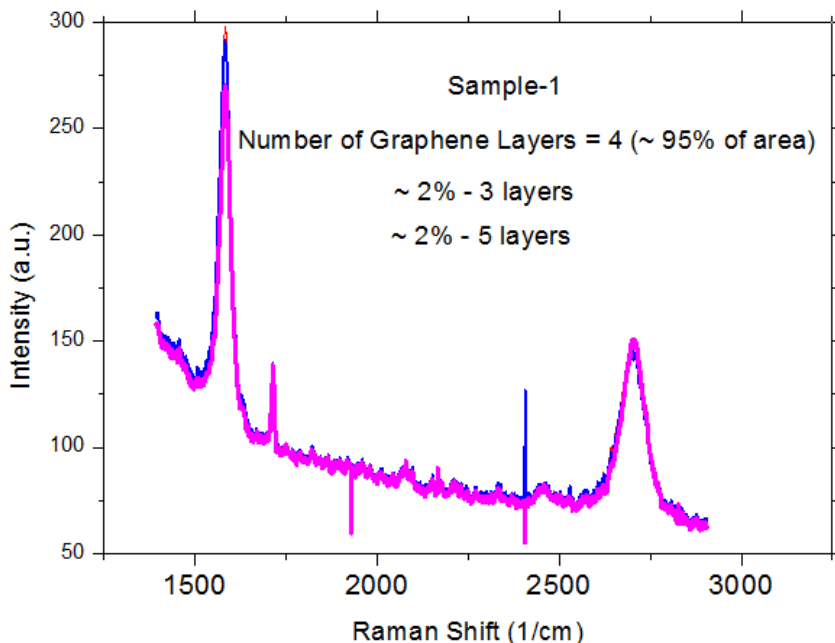
Рис. 1. Рамановский спектр исследуемого образца
