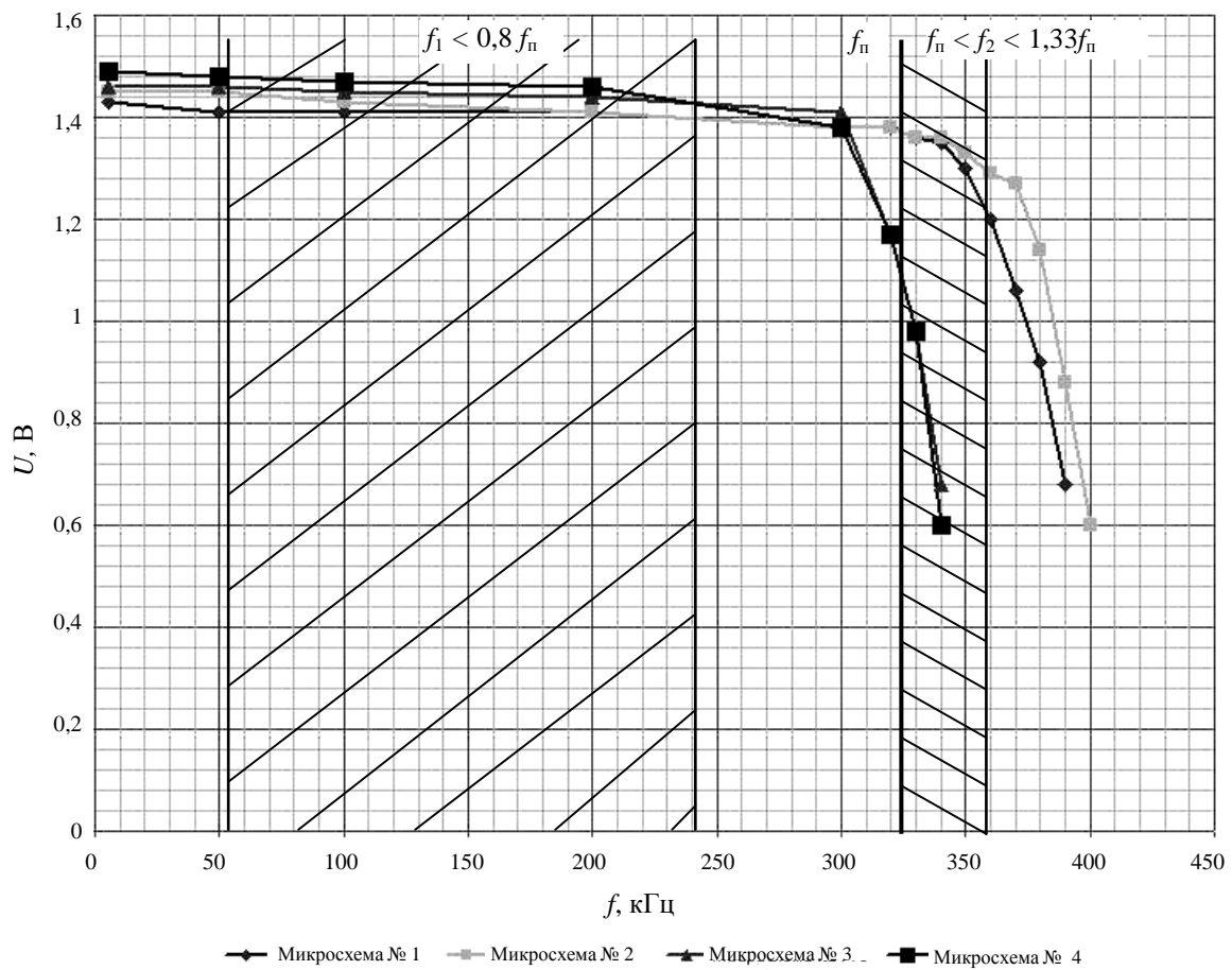
Рис. 1. Зависимость критических питающих напряжений от частоты тестирования интегральных схем
