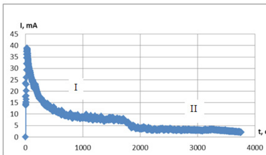
Рис. 1. Вольт-временная характеристика анодирования тонкой фольги (10 мкм) алюминия
