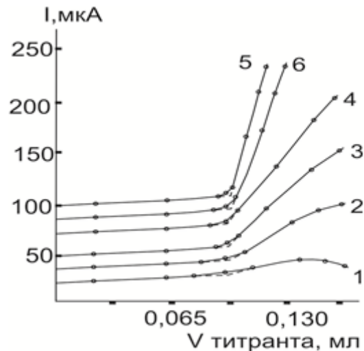
Рис. 1. Влияние напряжения на форму кривых АТ палладия (II) раствором ТАА на фоне 0,15 М по нитрату лития в уксусной кислоте. Величина напряжения, В: 1 — 0,10; 2 — 0,30; 3 — 0,50; 4 — 0,70; 5 — 0,90; 6 — 1,1
