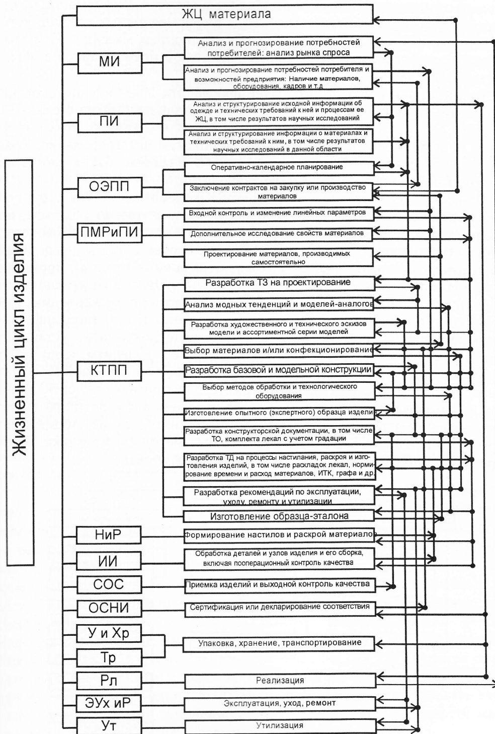
Рис. 2. Модель информационного взаимодействия подсистем ЖЦ швейных изделий
