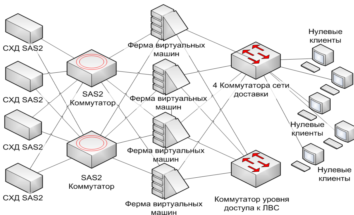
Рисунок 2 – Сеть виртуальных рабочих мест
