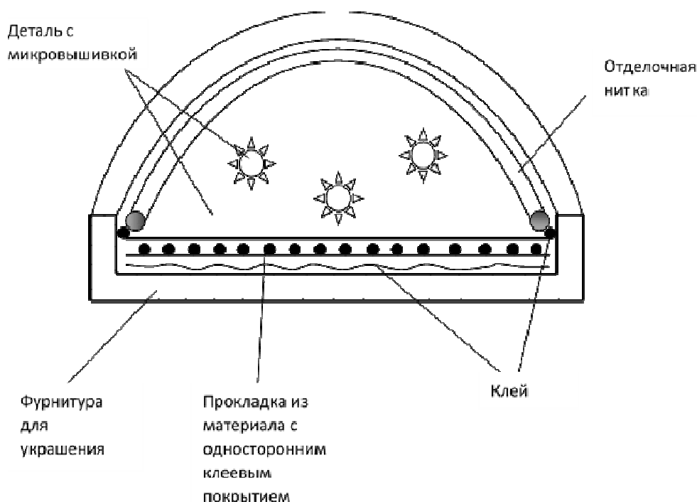
Рис. 4. Схема предлагаемого способа изготовления текстильной вставки с микровышивкой
