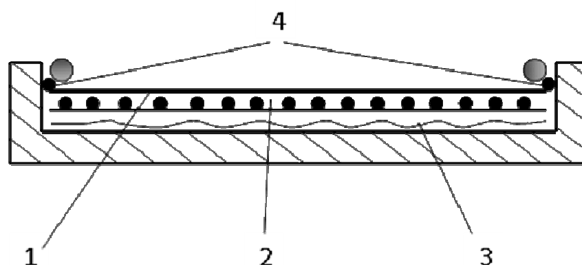
Рис. 5. Проекционная схема способа микровышивки крестиком на детали из основного материала – ткани равномерного переплетения для вышивки
