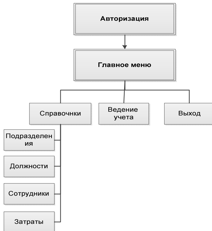
Рис. 2. Сценарий диалога системы
