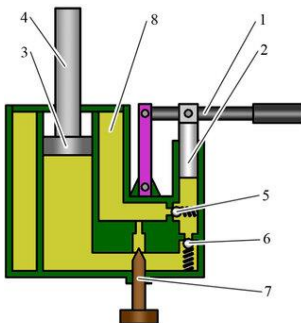
Рис. 3. Схема гидравлического домкрата
