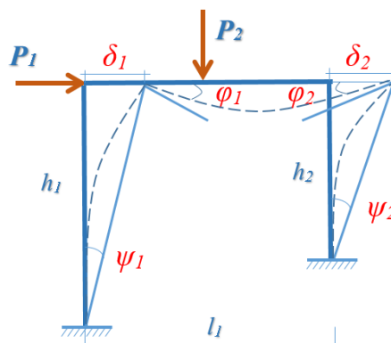
Рис.1. Деформированная статически неопределимая рама
