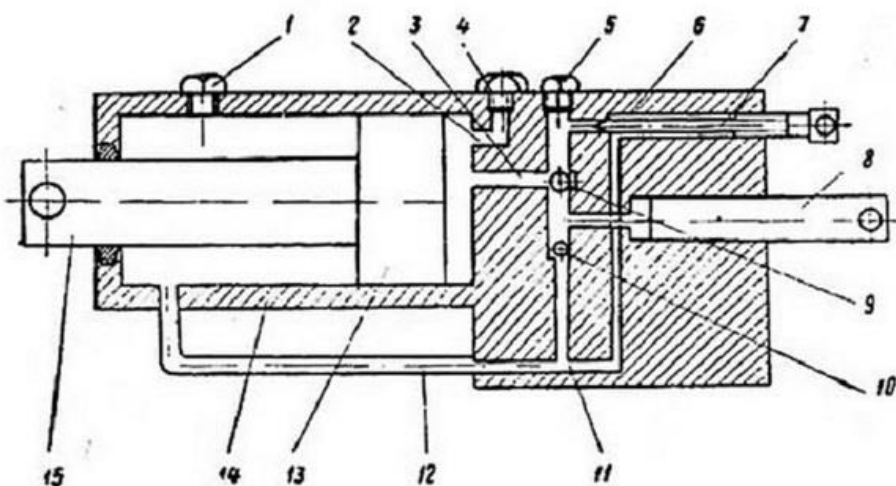
Домкрат гидравлический парковый:
