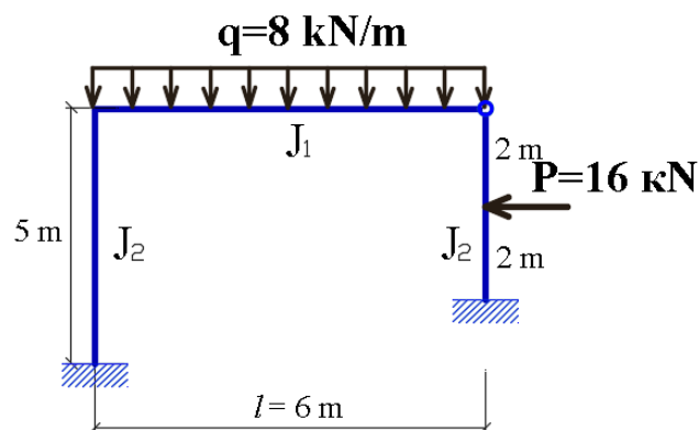
Рис. 2. Заданная схема
