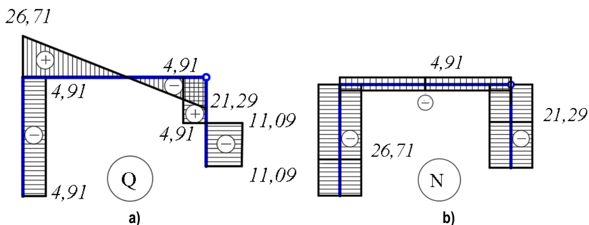
Рис. 6. Эпюры поперечной силы (а) и продольной силы (б)
