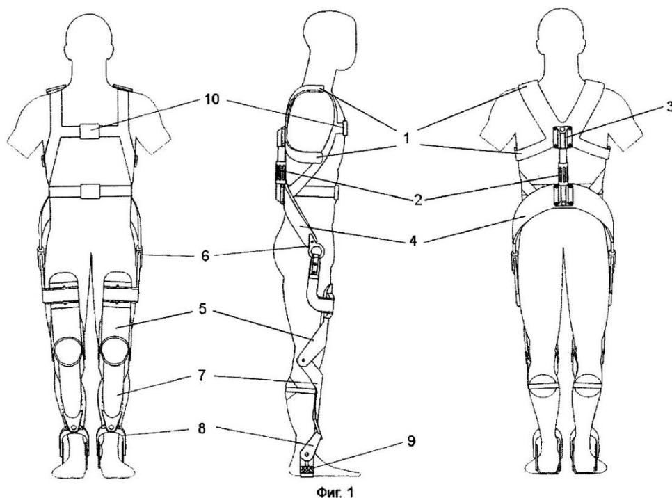
Рис. 1. Эскиз пассивного экзоскелета
