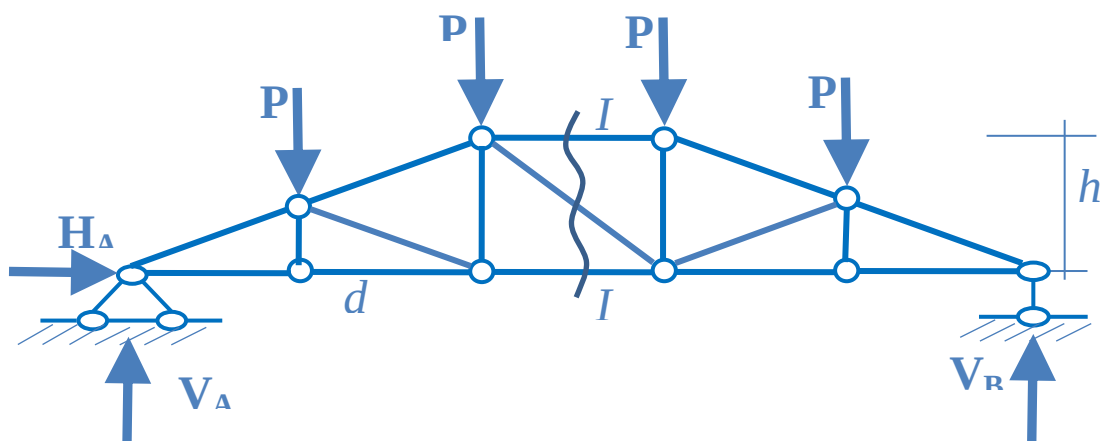
Рис. 2. Плоская статическая определимая ферма
