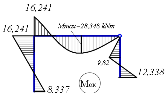
Рис. 5. Окончательная эпюра изгибающих моментов
