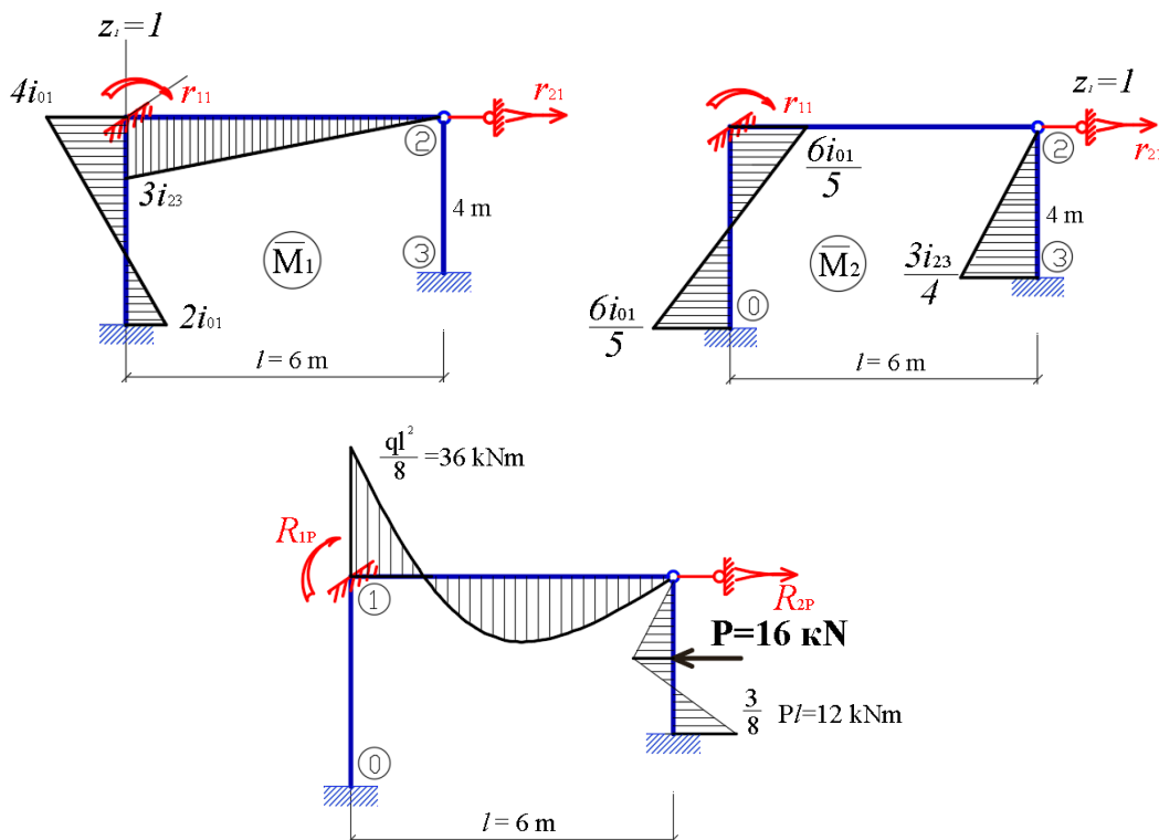
Рис. 4. Единичные и грузовые эпюры
