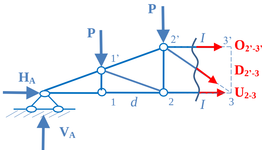
Рис. 3. I-I Сечение фермы
