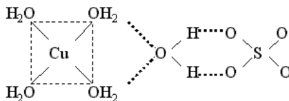
Рисунок 1 – Структура сульфата меди пятиводного
