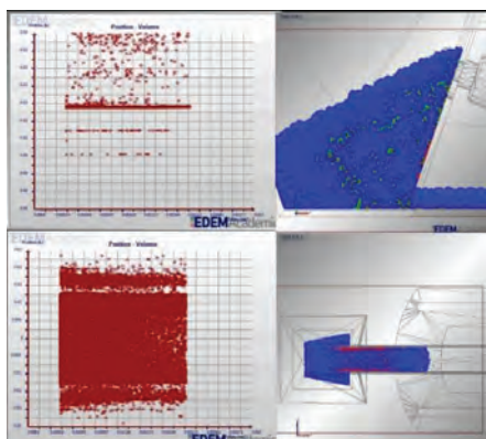
Рис. 1. Моделирование процесса вибротранспортирования в программе EDEM (DEM Solutions)
