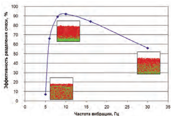
Рис. 4. Зависимость эффективности разделения частиц двухкомпонентной смеси от частоты вибрации при фиксированной амплитуде
