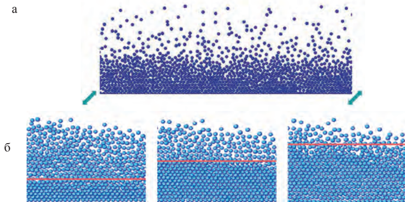
Рис. 2. Вибрационное транспортирование
