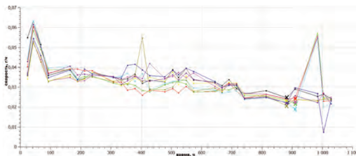
Рисунок 9 – Зависимость скорости испарения воды от времени для растворов \text{CuSO}_4 \cdot 5\text{H}_2\text{O}
