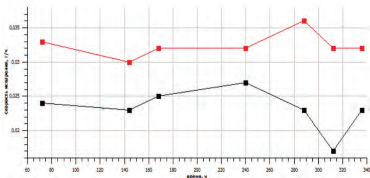
Рисунок 10 – Скорости испарения воды из контрольных растворов второй серии опыта - ■ – NiSO 4 ·7H 2 O; ■ – CuSO 4 ·5H 2 O
