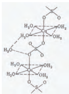
Рисунок 2 – Пространственная структура сульфата меди пятиводного
