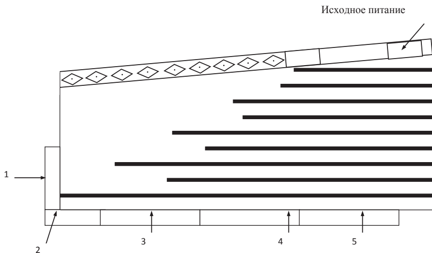
Рис. 1. Схема разделения на концентрационном столе.
