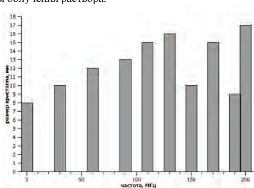
Рисунок 5 – Зависимость размера кристалла \text{CuSO}_4 \cdot 5\text{H}_2\text{O} от частоты облученной воды
