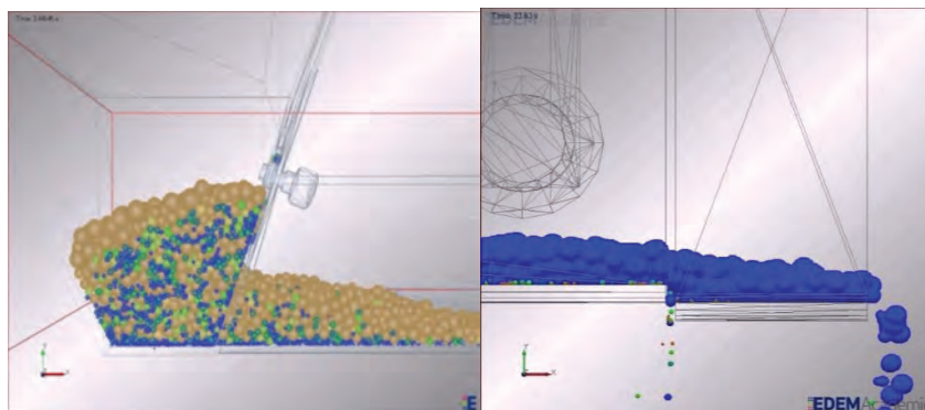
Рис. 5. Модель вибрационно-сегрегационного классификатора с щелевым отверстием
