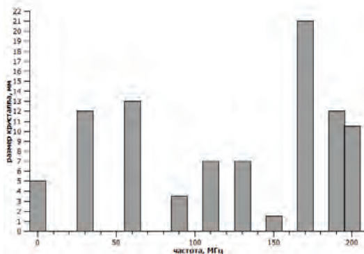
Рисунок 4 – Зависимость размера кристалла NiSO 4 ·7H 2 O от частоты облученной воды
