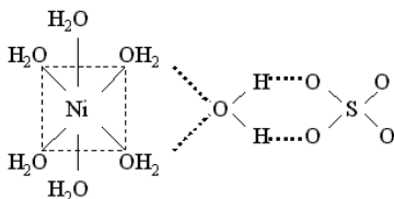
Рисунок 3 – Структура сульфата никеля семиводного
