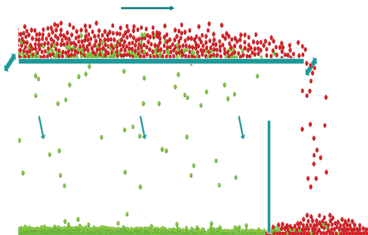
Рис. 3. Установившийся процесс грохочения смоделированный в программе EDEM (DEM Solutions Ltd.)
