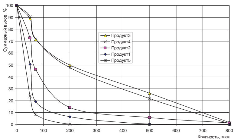
Рис. 2 Суммарный выход по пяти продуктам
