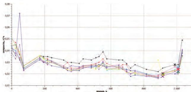
Рисунок 8 – Зависимость скорости испарения воды от времени для растворов \text{NiSO}_4 \cdot 7\text{H}_2\text{O}
