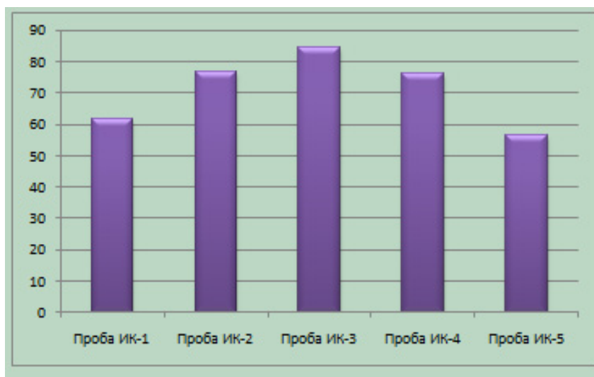
Рисунок 2 – Степень защиты ингибиторами ИК-1 - ИК-5, %
