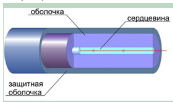
Рисунок 3 – Одномодовое ОВ
