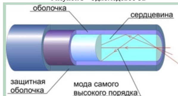
Рисунок 4 – Многомодовое ОВ
