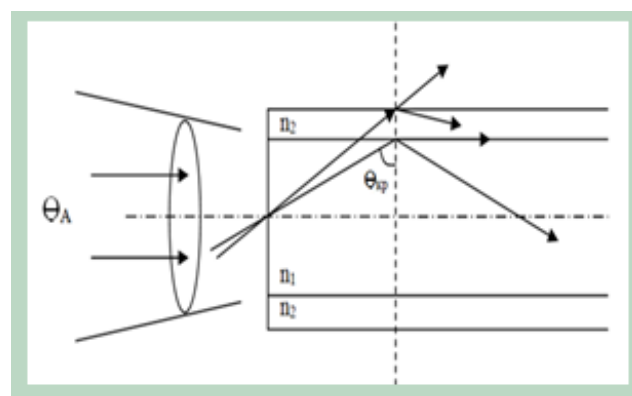
Рисунок 2 – Полное внутреннее отражение
